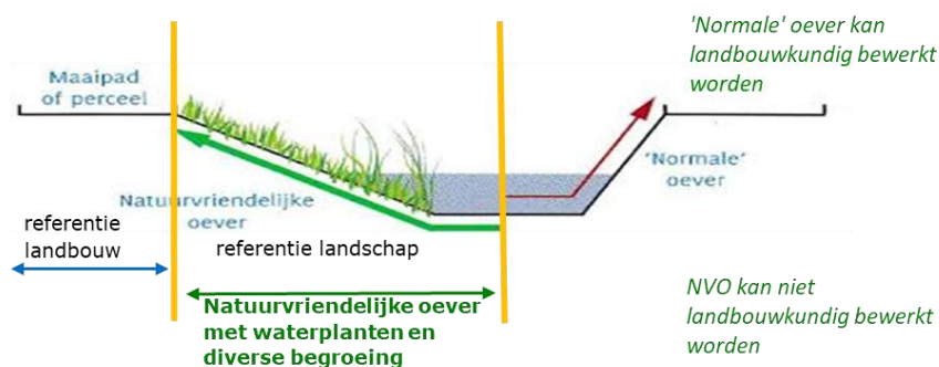
Figuur 1: Tekening natuurvriendelijke oever (NVO) © BoerenNatuur.
